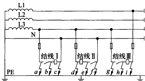
图1 控制回路结线示例图
